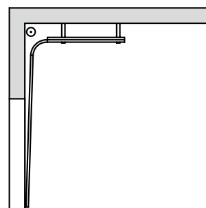
Druh kování H Výše vedené Kování na kolejnici
